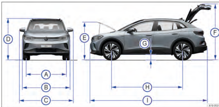
Рис. 206 Габаритные размеры.
