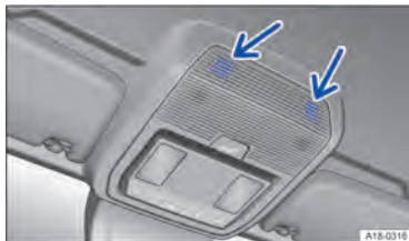
Рис. 64 В потолочной консоли: датчики система заднего наблюдения (стрелки).
