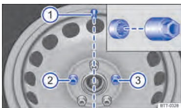
Рис. 192 Замена колеса: вентиль шины 1 также расположение противогононного болта колеса 2 или же 3.
